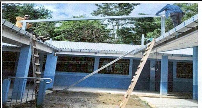
Foto 4: COLOCACIÓN DE ESTRUCTURA METALICA PARA ENTECHADO GALVANIZADA 4X4X6 CHAPA 16 DE 5X10 METROS, SUSTITUCIÓN DE MEJORAS DE LOS SERVICIOS SANITARIOS
