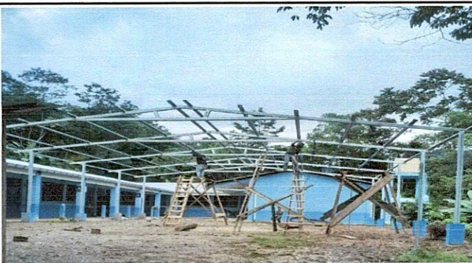
Foto 3: COLOCACIÓN DE COSTANERAS 2X4X6 CHAPA 16 PARA LA COLOCACIÓN DE LÁMINAS GALVANIZADAS
