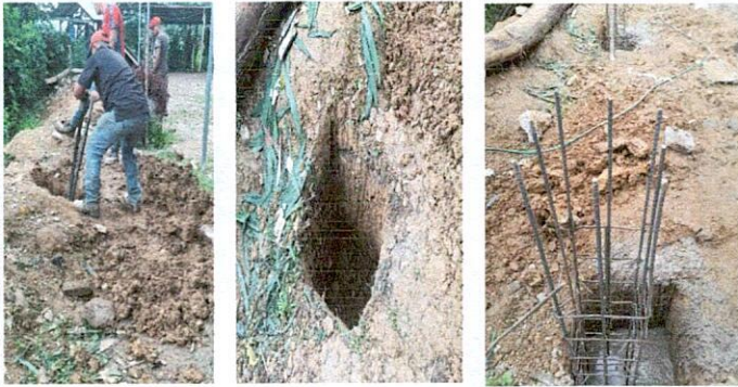
Foto1: INICIO DEL TRABAJO CON PERFORACIÓN PARA FUNDIR BASES DE CONCRETO Y ESTRUCTURA METAL GALVANIZADA
